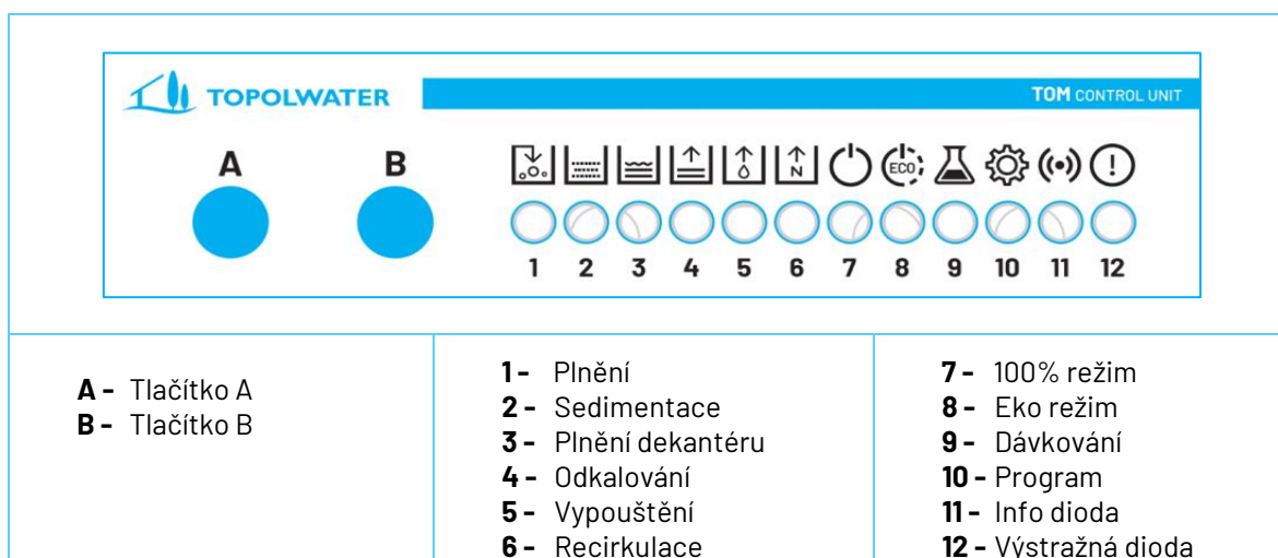
Obrázek 6: Popis řídicího panelu
