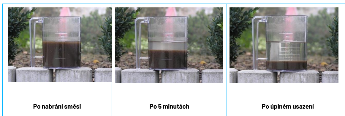
Obrázek 11: Kontrola množství kalu v aktivaci
