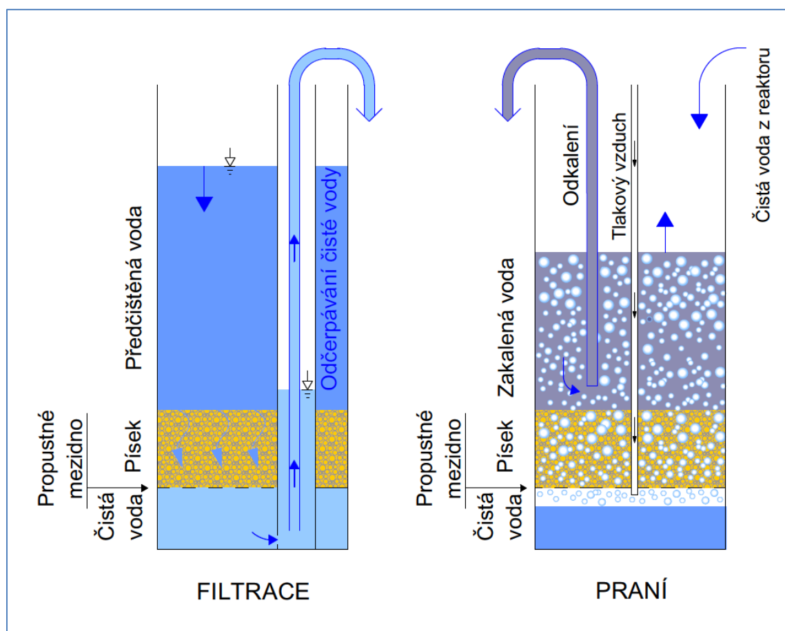
Obrázek 2: Princip funkce pískového filtru
